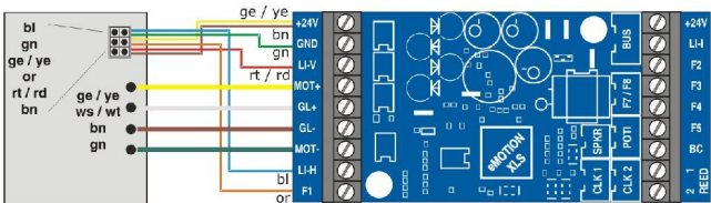
Abbildung 7: Einbau in Lok mit LGB® Dekoder-Schnittstelle
