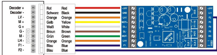
Abbildung 8: Verwendung des Schnittstellenkabels an LGB® DCC Schnittstelle
