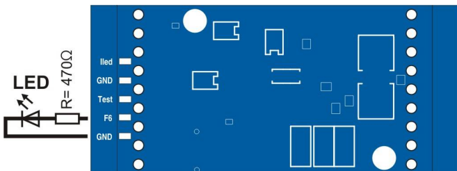
Abbildung 11: Licht und Funktionsausgang Unterseite und dessen Verschaltung
