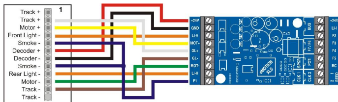
Abbildung 9: Verwendung des Schnittstellenkabels an einer Aristocraft® DCC Schnittstelle
