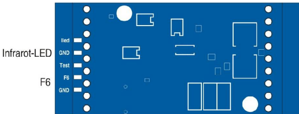
Abbildung 6: Belegung der Anschlusslötkontakte (Unterseite)
