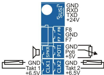
Abbildung 2: Belegung der Anschlussbuchsen Massoth-Bus
