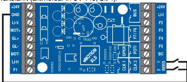
Abbildung 12: Anschluss der Reedkontakte
