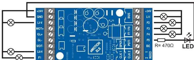
Abbildung 10: Licht und Funktionsausgänge und deren Verschaltung
