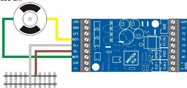
Abbildung 4: Einbau des eMOTION XLS
