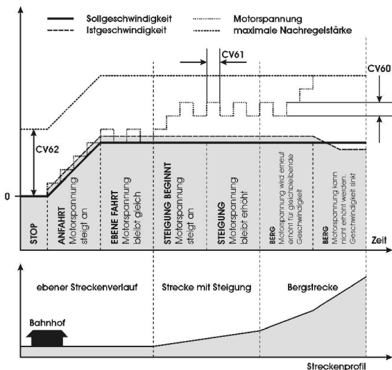
Abbildung 14: Funktionsweise der Lastregelung
