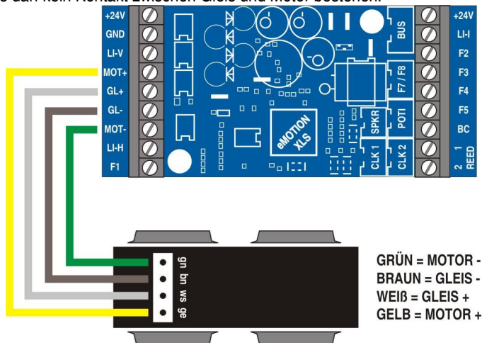
Abbildung 5: Anschluss an LGB® Getriebe
