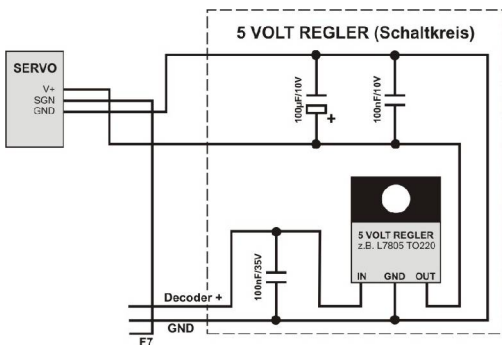
Abbildung 15: 5 V Regler für Servomotor
